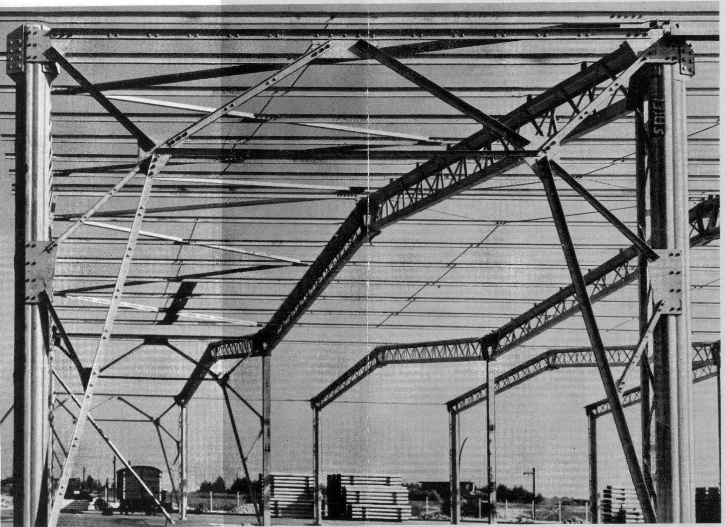
Hallenbau aus vorfabrizierten Stahlbindern
